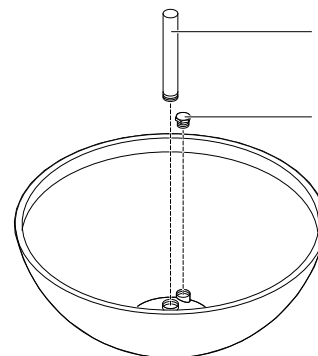
84169 Kupferschale Rund 90
