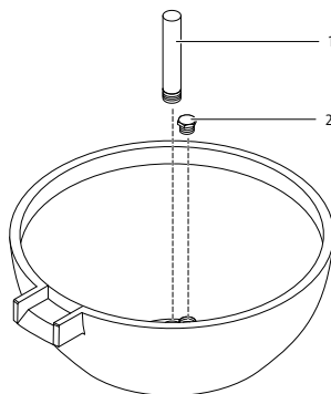
84168 Kupferschale Rund 75
